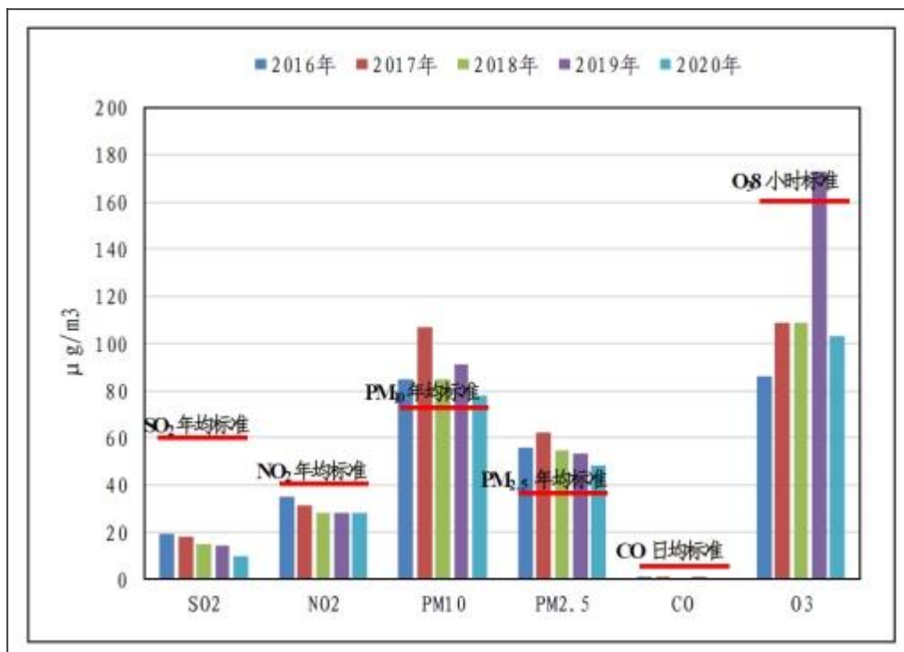
图 1 2016-2020 年淮南市空气环境质量变化情况(其中 CO 单位：mg/m 3 )
