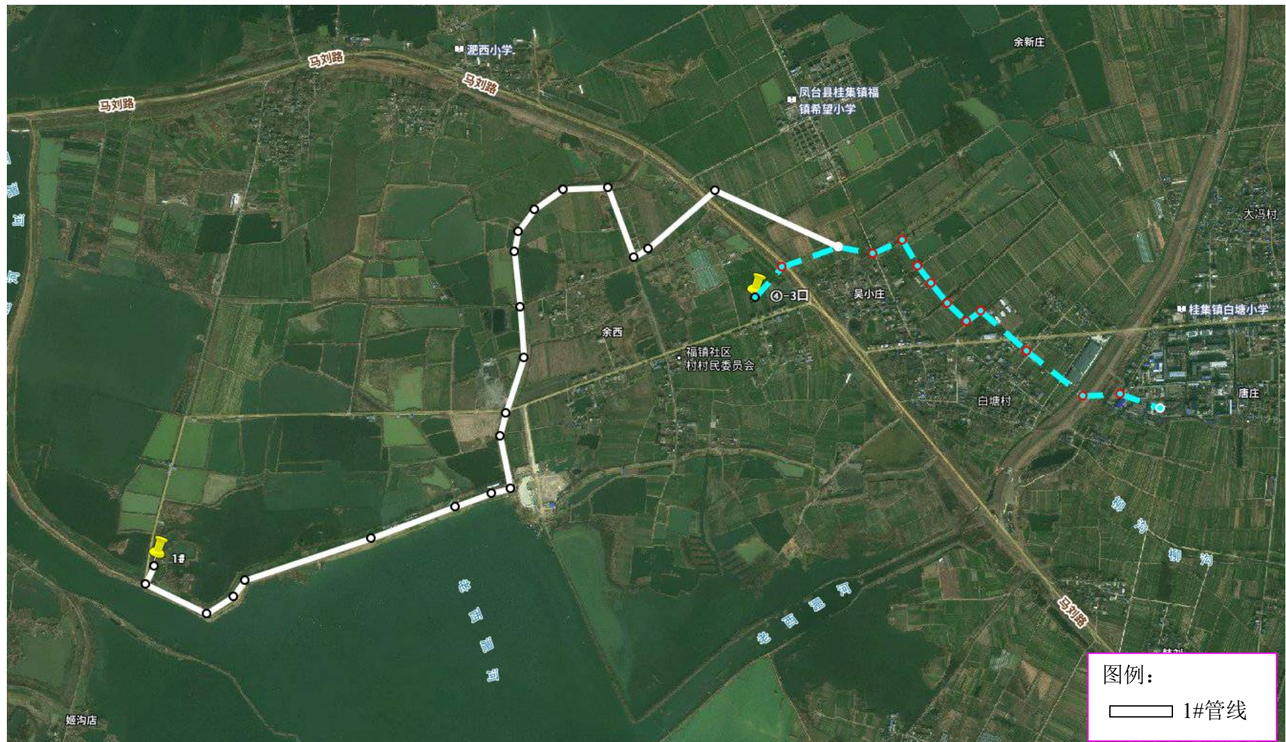
图 3.2-11 1#井场管路路线示意图
