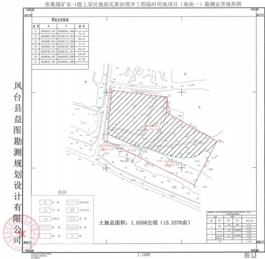
图 3.2-4 井场 1 临时用地勘测定界图
