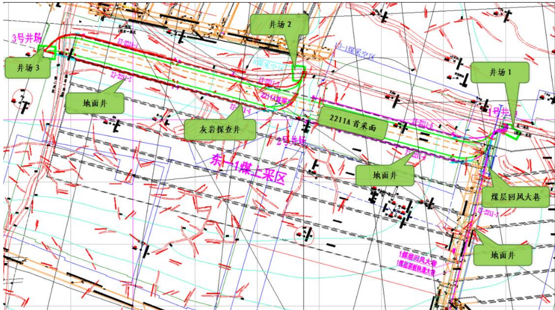
图 3.2-10 采区地面瓦斯区域治理井井场布置图
