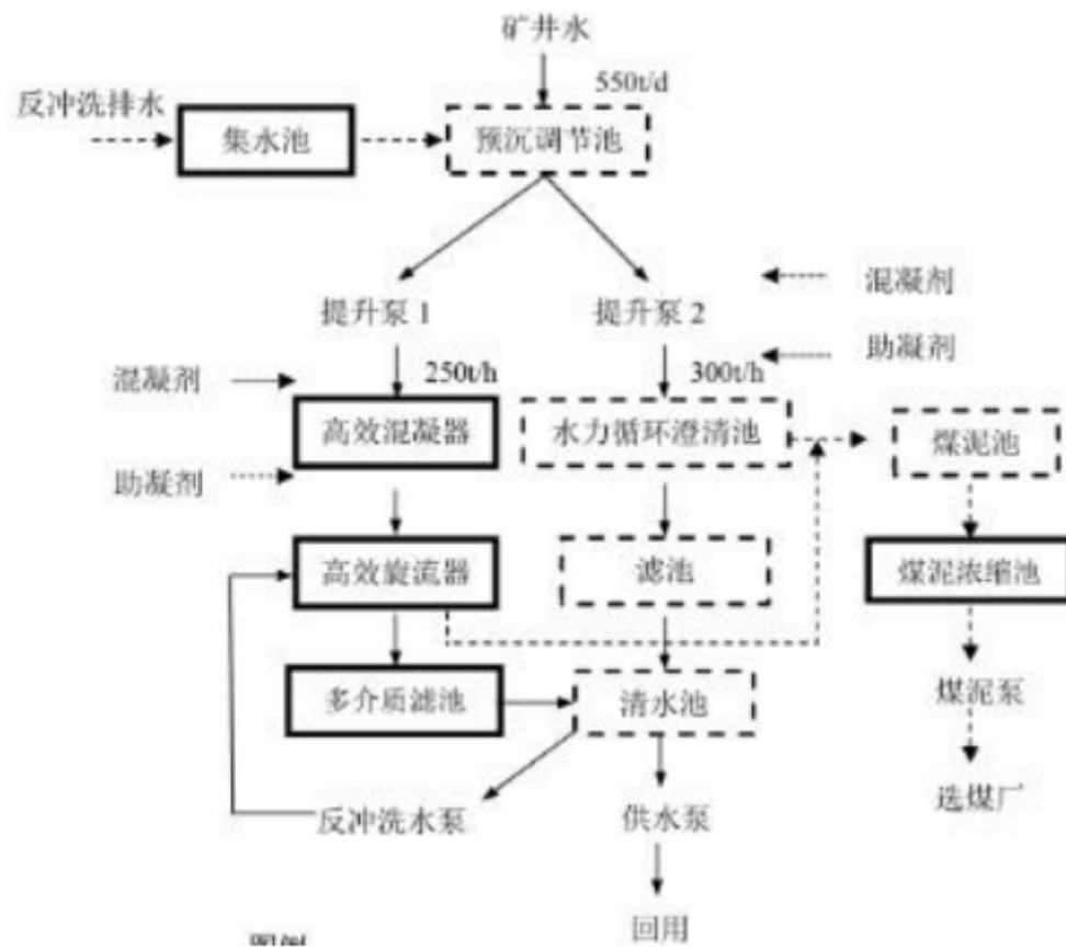
图 7.2-1 张集矿井中央区、北区污水处理站工艺流程图
