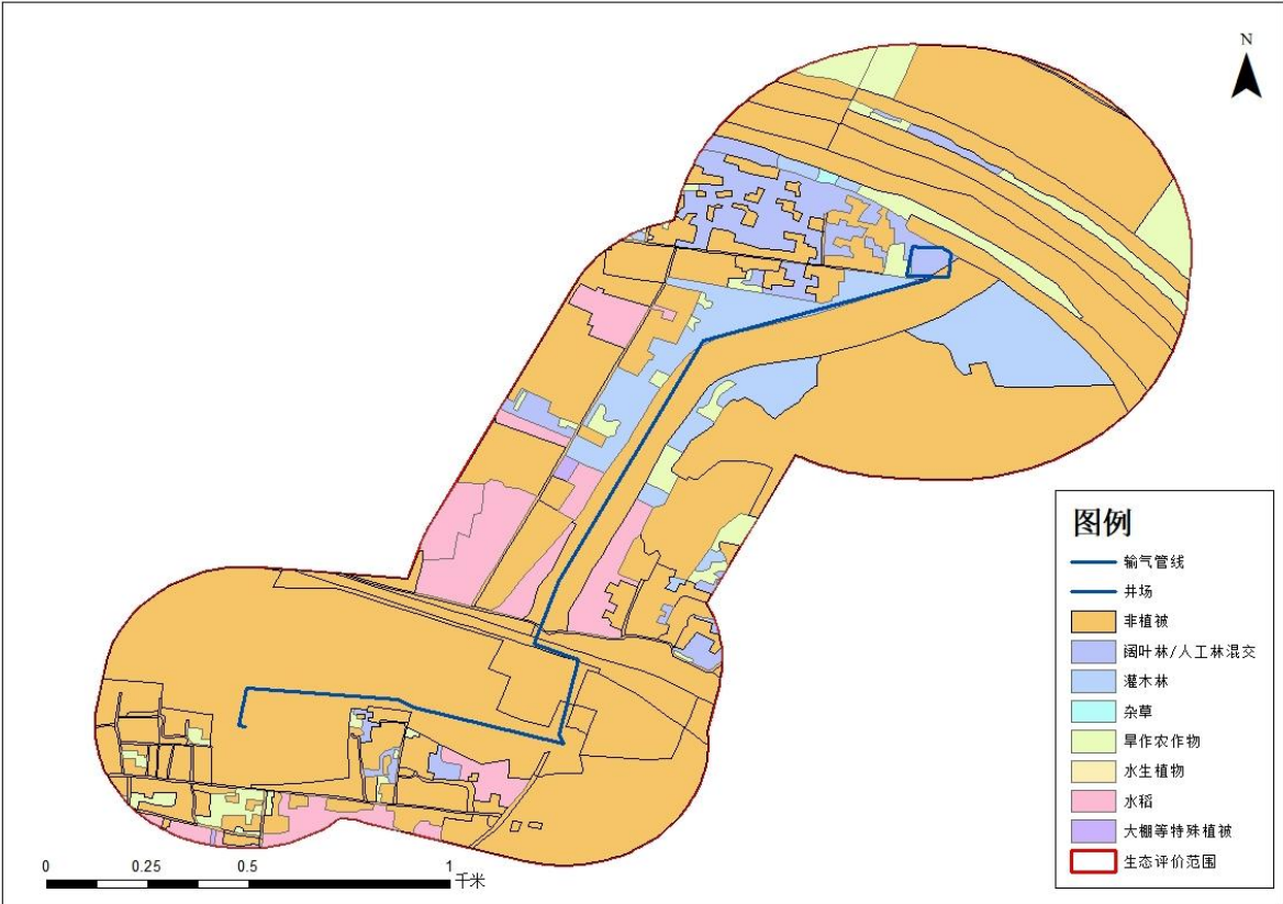
图 4.2.5-9 本项目评价区植被类型图
