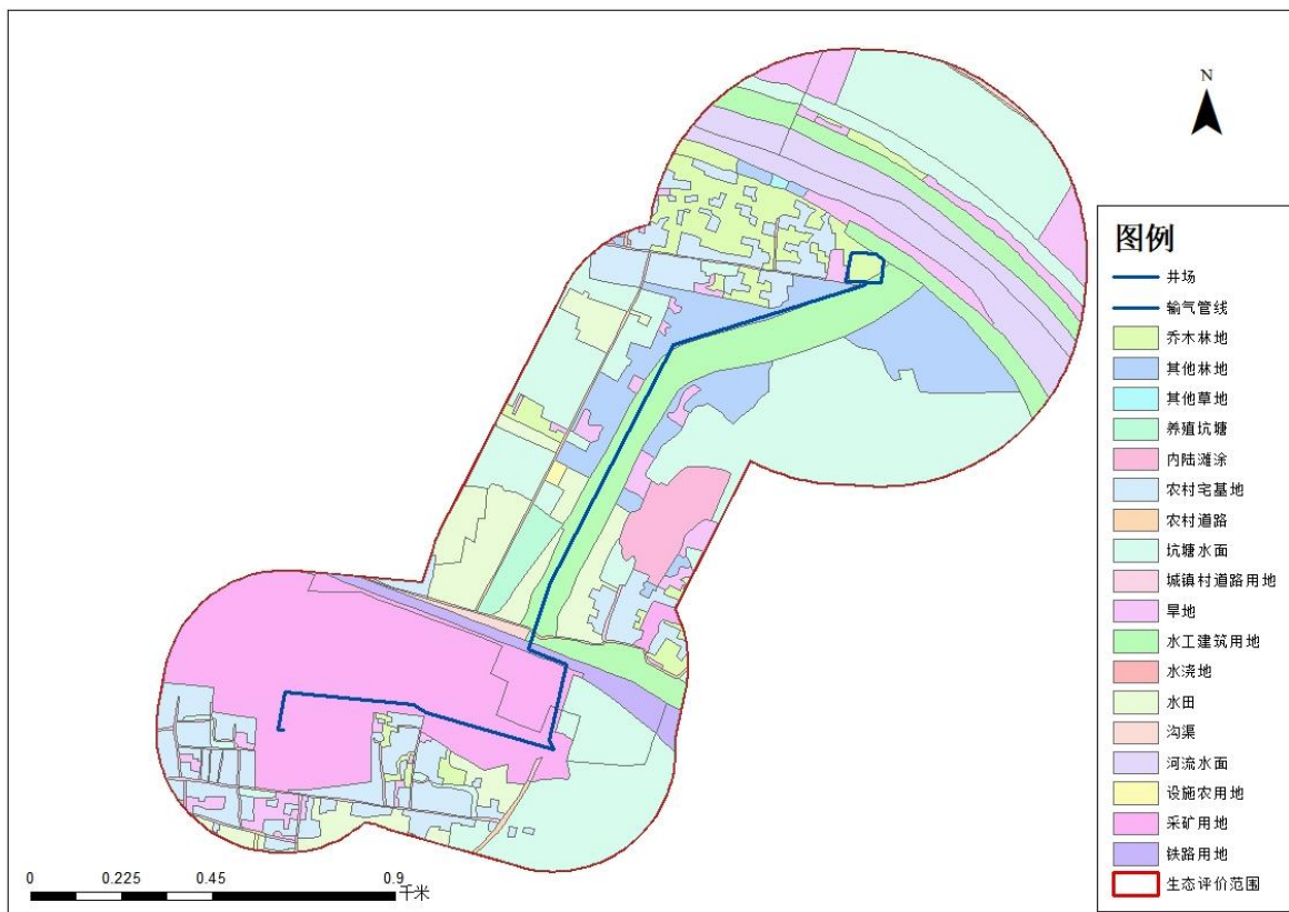
图 4.2.5-10 本项目生态评价范围土地利用现状图
