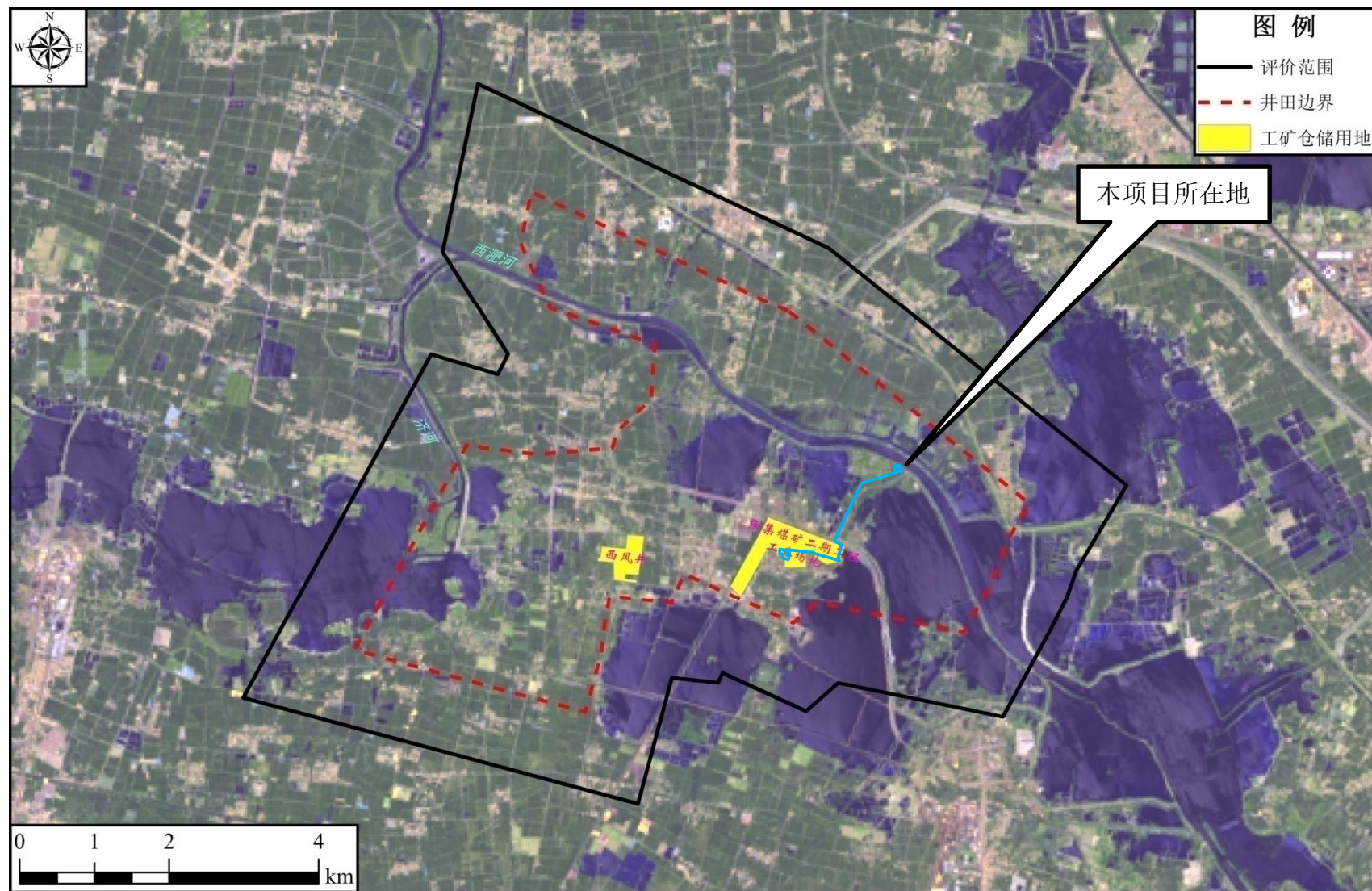
图 4.2.5-1 卫星遥感影像图
