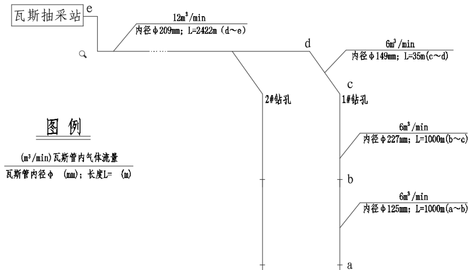
图 3.1-1 瓦斯管路系统阻力计算示意图
