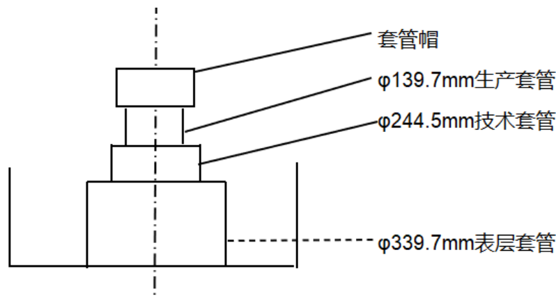
图 3.3-3 水平井完井井口示意图
