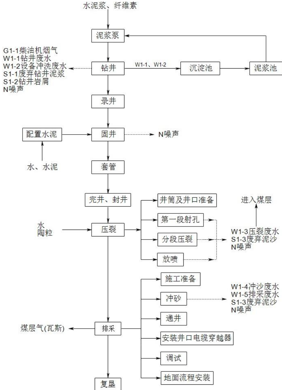
图 3.3-1 瓦斯治理井工程施工工艺与产污环节流程
