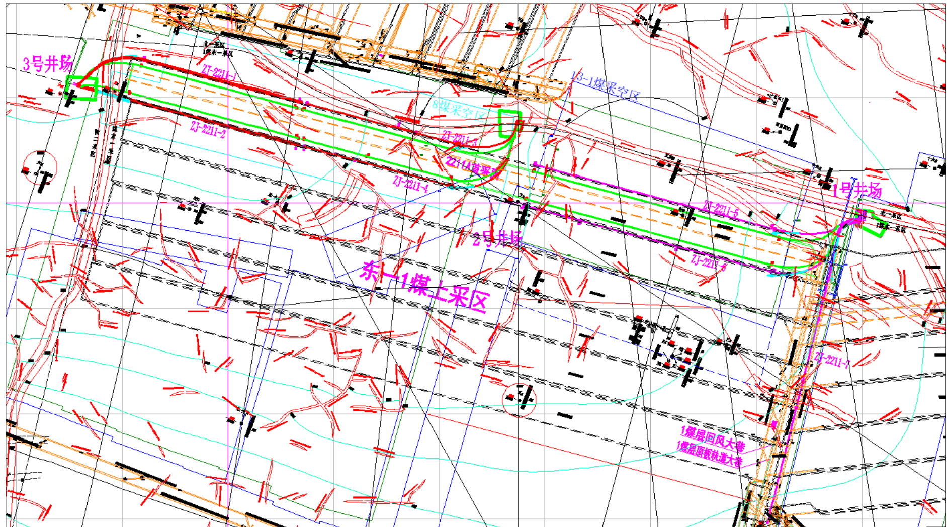
图 3.2-3 张集煤矿东—1煤上采区地面瓦斯治理井平面布置图
