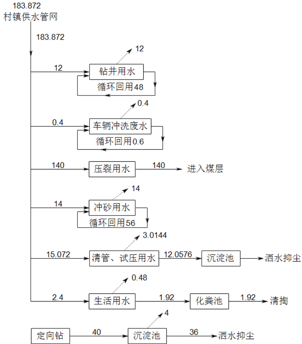
图 3.4-1 施工期水平衡(m³/d)
