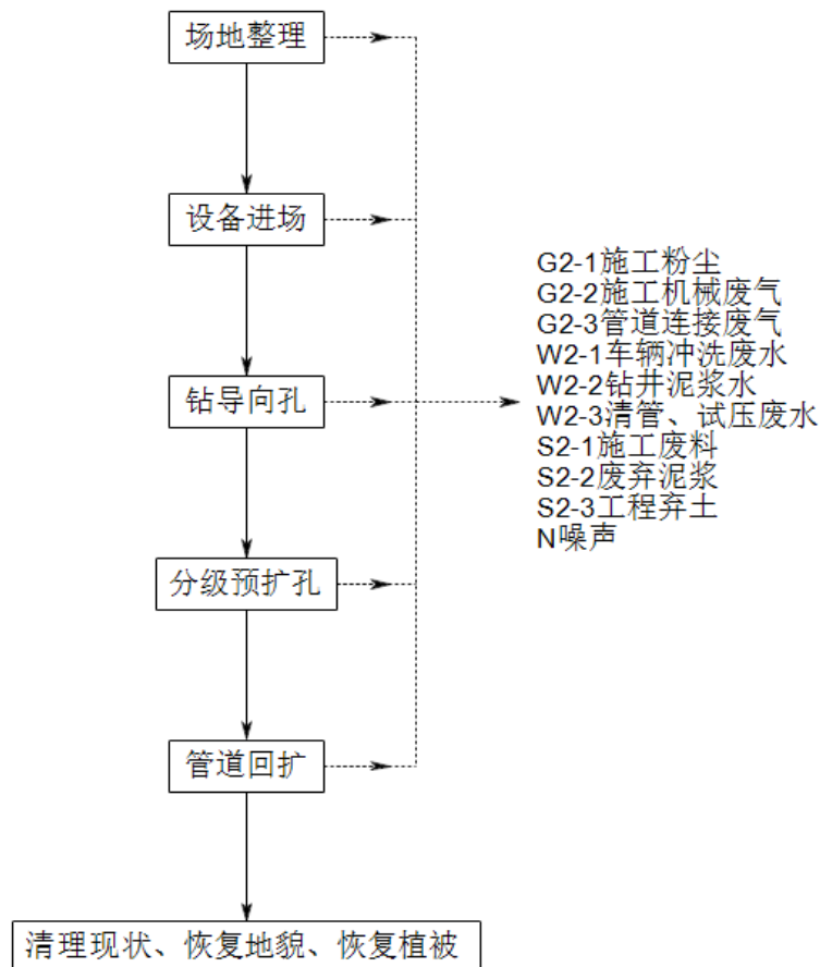
图 3.3-4 定向钻施工工艺流程及产污环节示意图
