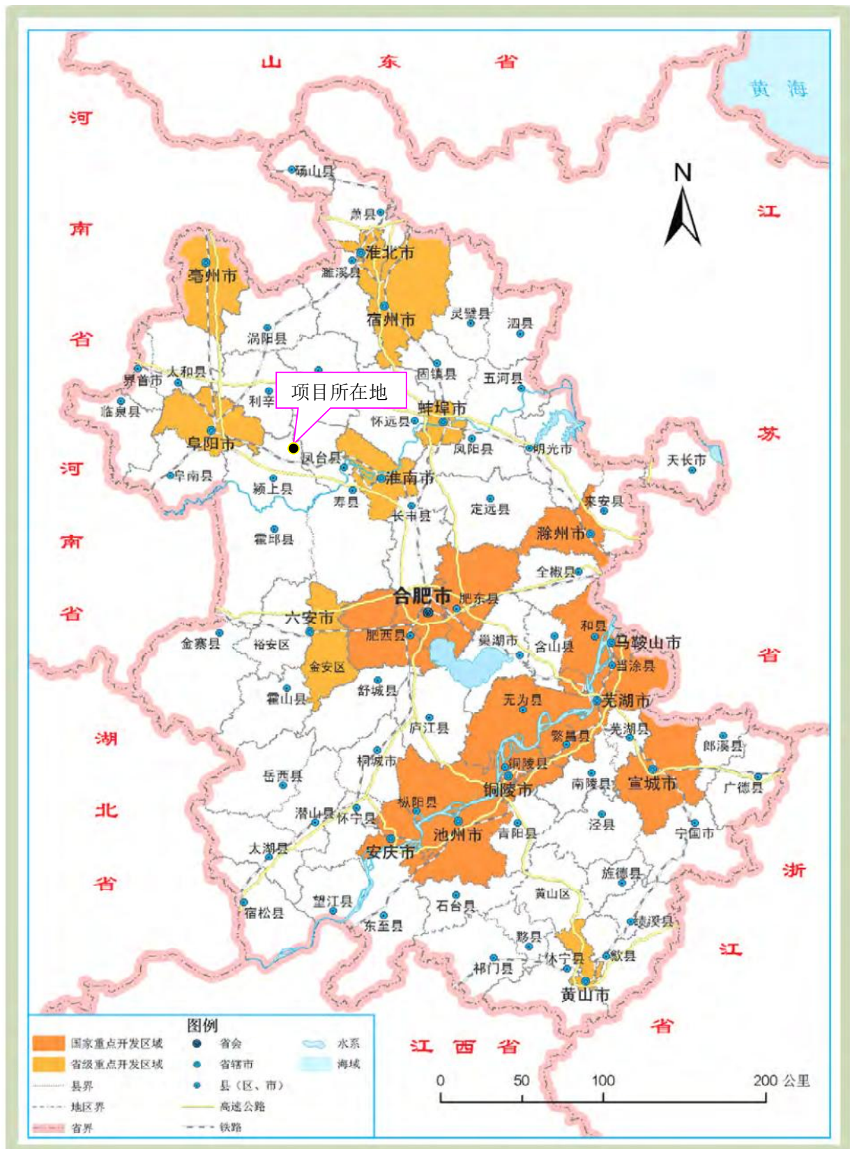
图 2.6-8 安徽省重点开发区域分布图
