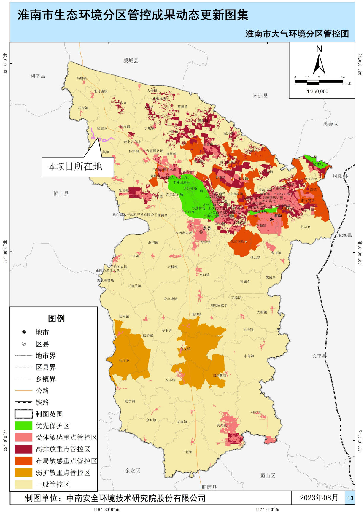
图 2.6-5 淮南市大气环境分区管控图
