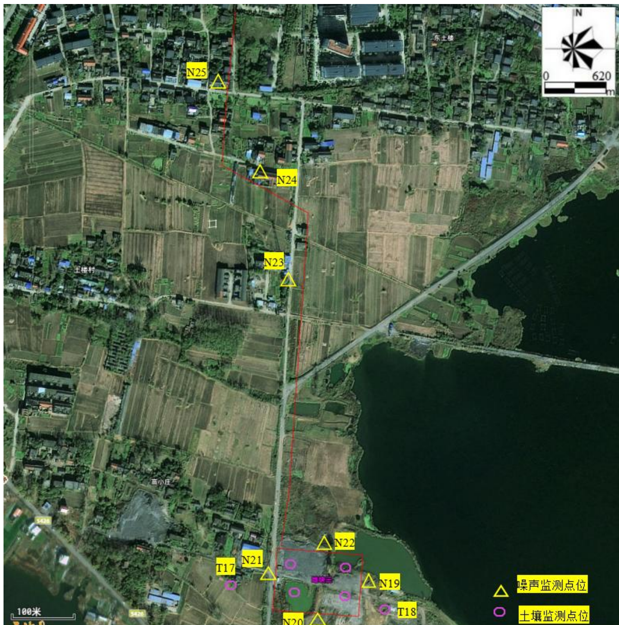
图 4.2-4 3#井场及管线声环境监测、土壤环境监测点位图
