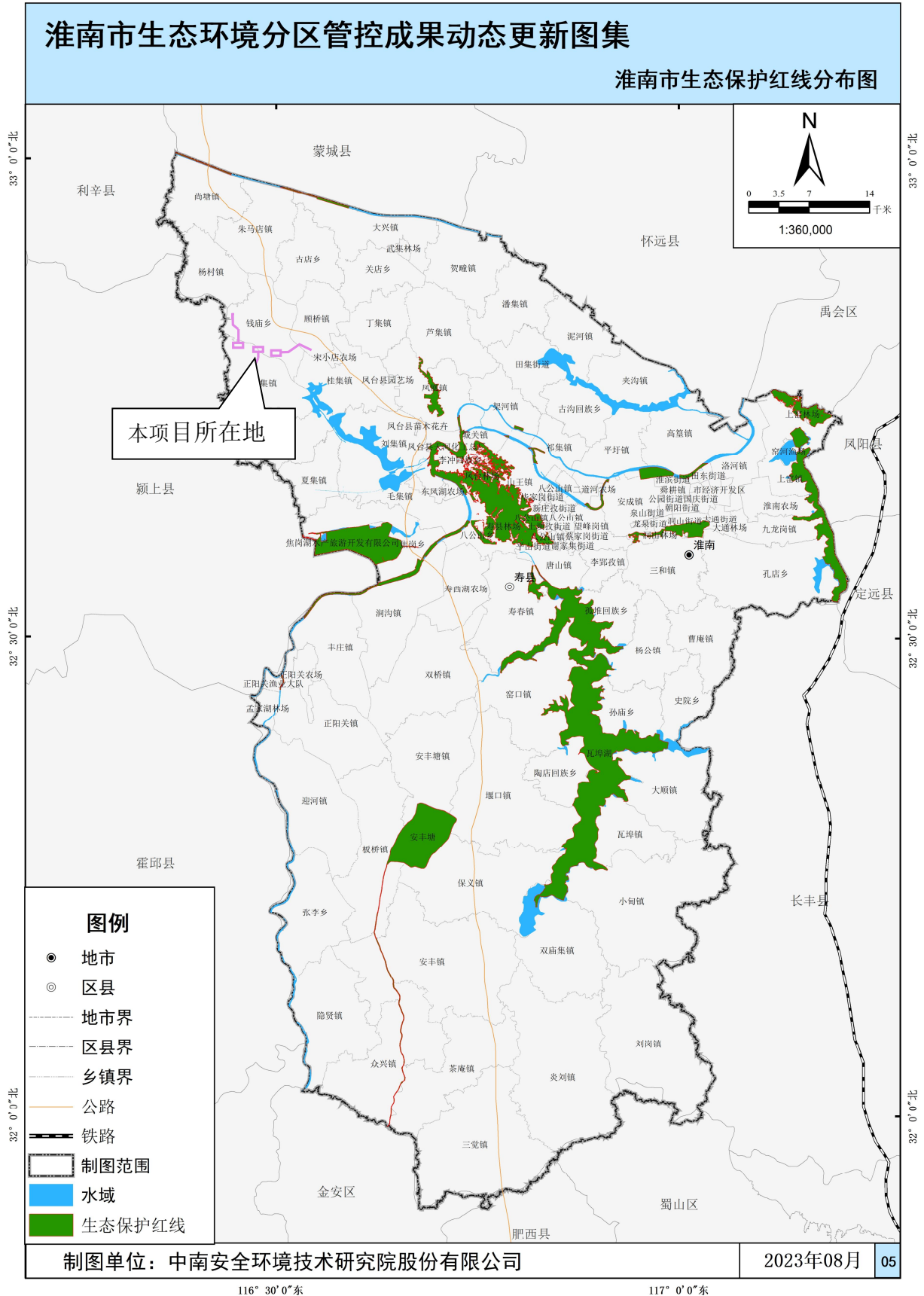
图 2.6-2 淮南市生态保护红线图
