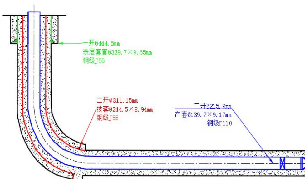
图 3.3-2 井身结构示意图
