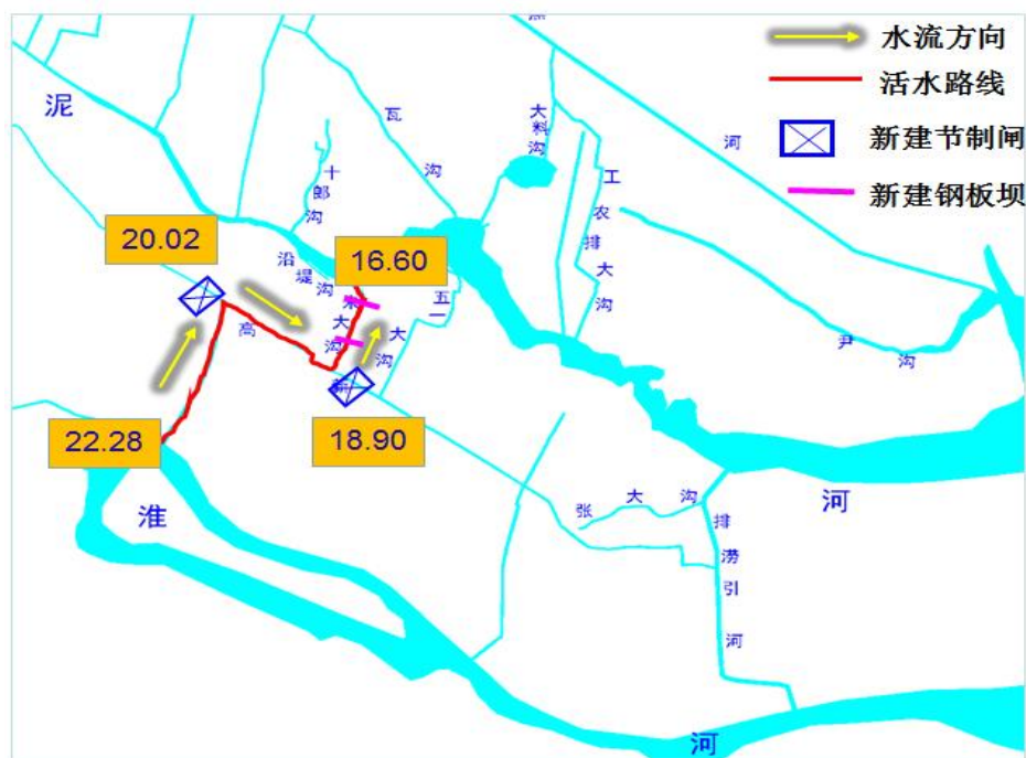
图 3.3.3-2 活水路线图
